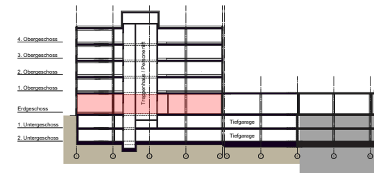
Schemaschnitt Hertistrasse 25
