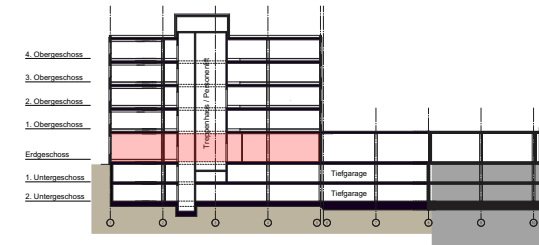
Schemaschnitt Hertistrasse 25
