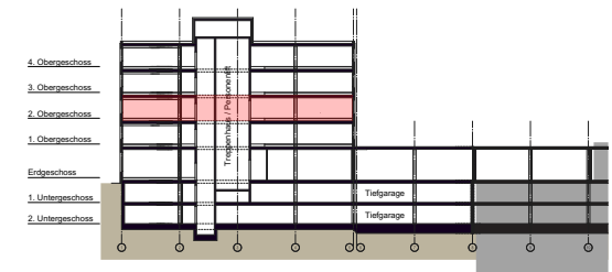
Schemaschnitt Hertistrasse 25
