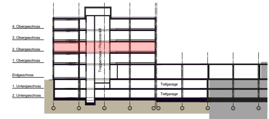
Schemaschnitt Hertistrasse 25
